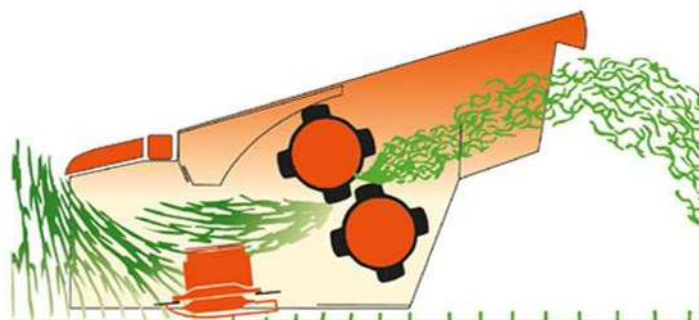
A felső henger előrébb van mint a hátsó, így a termés felfelé áramlik
